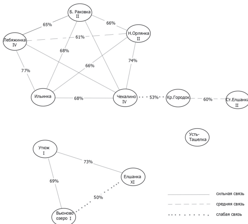
Рисунок 1 – Граф связей памятников елшанской культуры по мотивам орнамента
